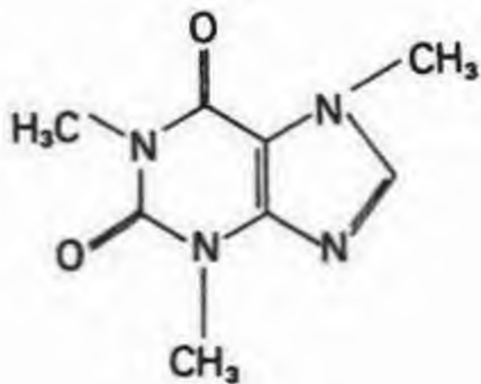
CAFFEINE
